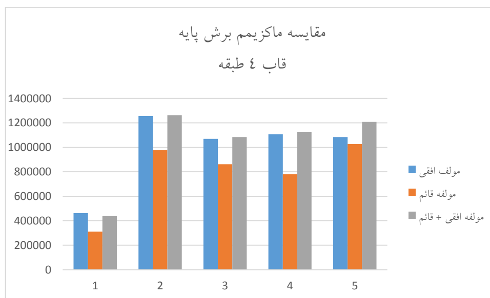
نمودار ۷- مقایسه ماکزیمم برش پایه قاب ۴ طبقه
