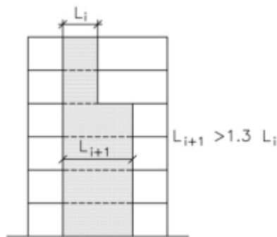
شکل ۶- نامنظمی در ارتفاع - هندسی [۴]
