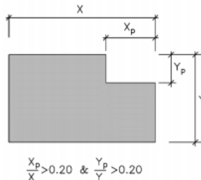
شکل ۱- نامنظمی در پلان - هندسی [۴]
