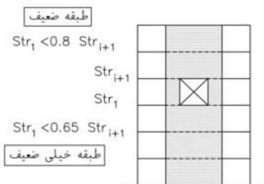
شکل ۹- نامنظمی در ارتفاع - مقاومت جانبی [۴]
