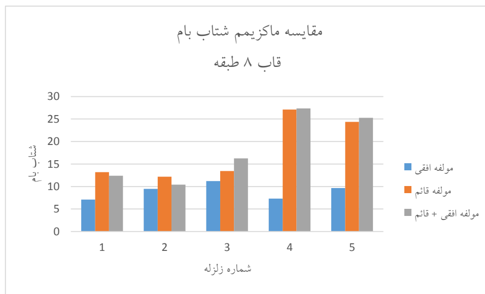
نمودار ۶- مقایسه ماکزیمم شتاب بام قاب ۸ طبقه
