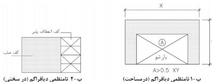
شکل ۳- نامنظمی در پلان - دیافراگم [۴]
