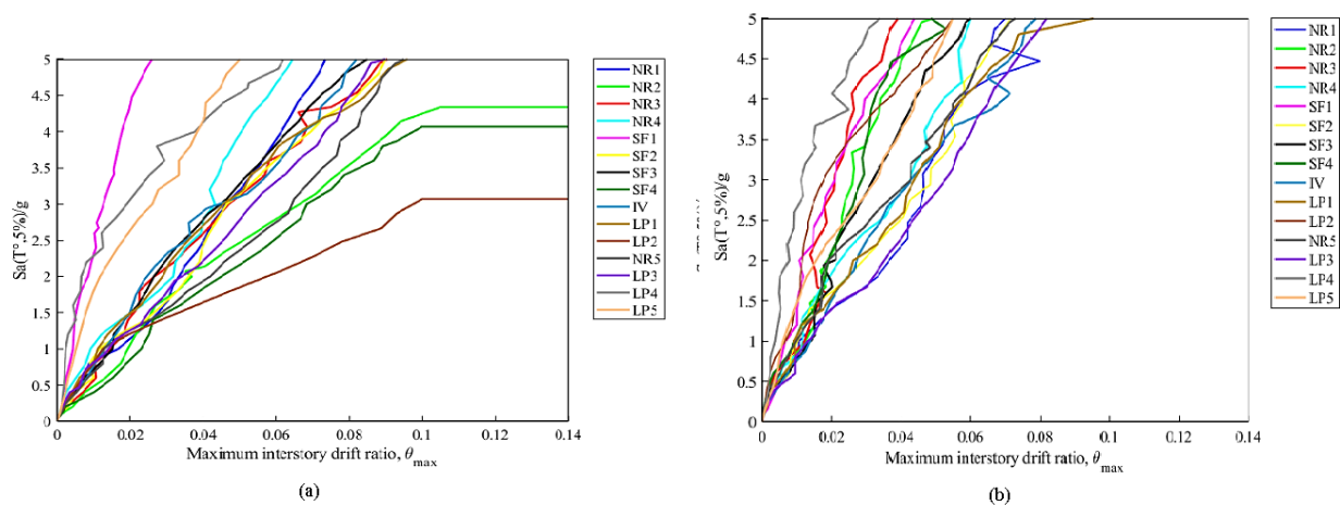
شکل ۳- منحنی های IDA قاب ۹ طبقه، a قاب SW9-1، b قاب SW9-2
