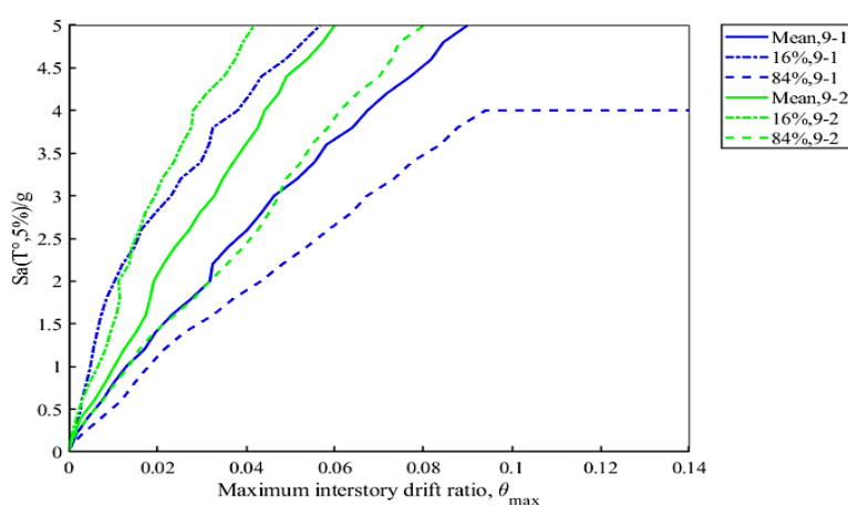
شکل ۷- خلاصه منحنی های IDA، قاب SW9-۱ و SW9-۲
