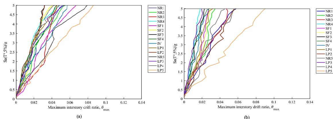
شکل ۲- منحنی های IDA قاب های ۶ طبقه، a قاب SW6-1، b قاب SW6-2
