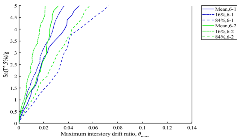
شکل ۶- خلاصه منحنی های IDA، قاب SW6-۱ و SW6-۲
