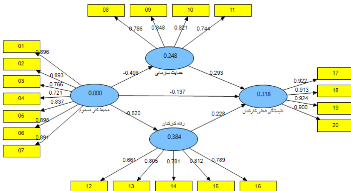
شکل ۴-۵: ضرایب تاثیر
